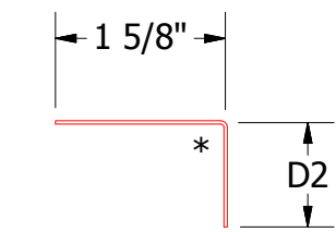
Angle Trim DWA680: D2=1" DSA680: D2=1 3/4"
