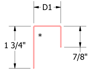
J Closure DWA270: D1= 1 1/8" DSA270: D1= 1 7/8"
