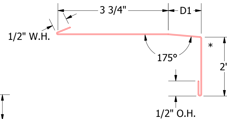
Window Sill Trim DWA670: D1= 1 1/8" DSA670: D1= 1 13/16"
