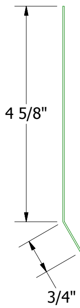
BGA369-Starter Cleat
